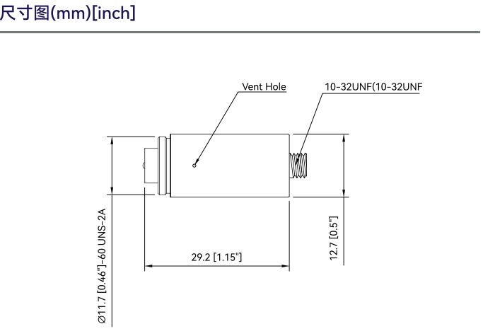
图1 CRY510B 前置放大器尺寸图
