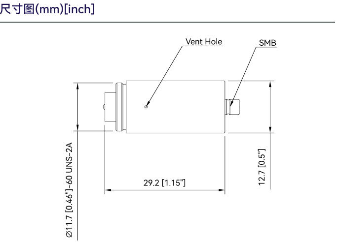
图1 CRY510 前置放大器尺寸图
