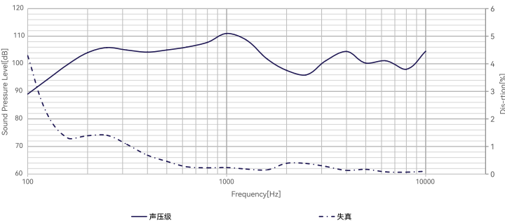
1 CRY605 仿真嘴典型频率响应和失真(25mm MRP)
