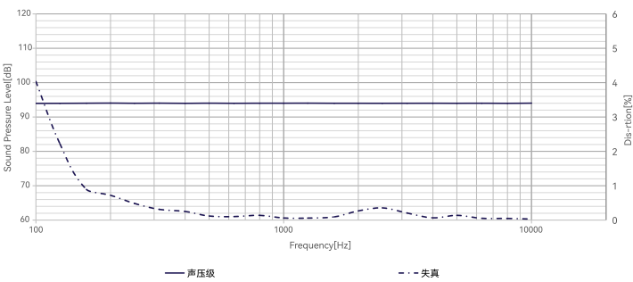
图2 CRY3602仿真嘴补偿后典型频响和94dB处的失真
