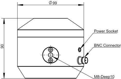
图3 CRY3602 仿真嘴尺寸图
