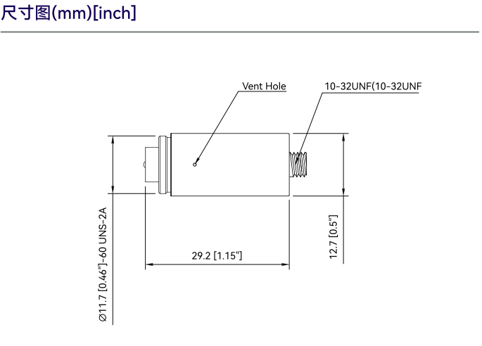
图1 CRY3503 前置放大器尺寸图
