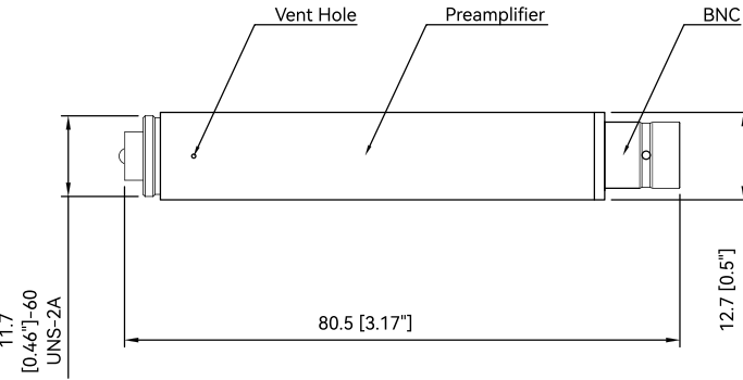
图1 CRY3501 前置放大器尺寸图
