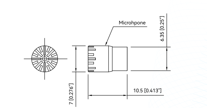
图1 CRY3485 测量传声器尺寸图
