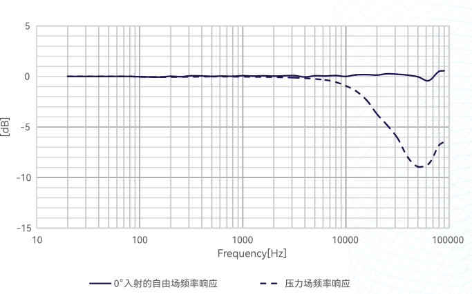
图2 CRY3485 测量传声器典型频响曲线
