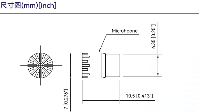
图1 CRY343 测量传声器尺寸图
