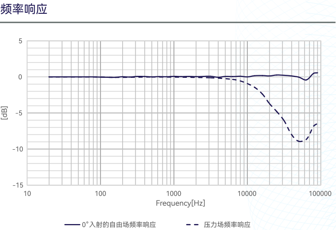
图2 CRY343 测量传声器典型频响曲线
