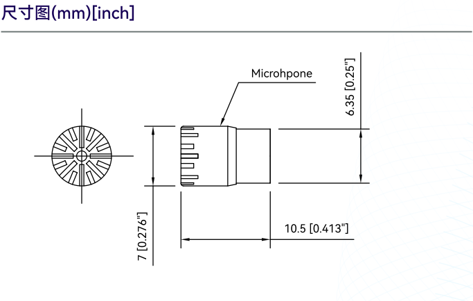
图1 CRY3406 测量传声器尺寸图
