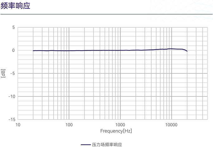
图2 CRY3406 测量传声器典型频响曲线
