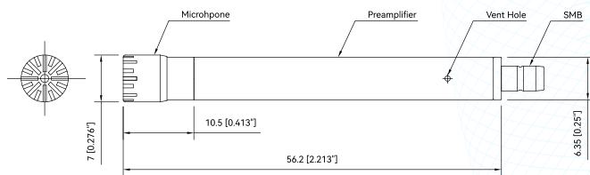
图2 CRY3406-S01 测量传声器套装尺寸图
