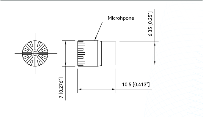
图1 CRY3402 测量传声器尺寸图
