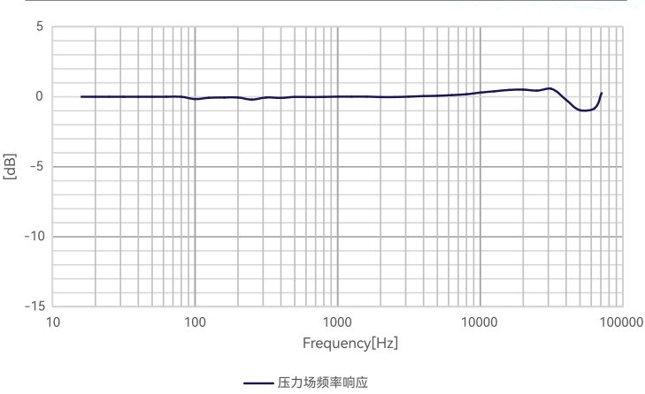
图2 CRY3402 测量传声器典型频响曲线
