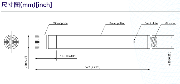
图2 CRY3402-S02 测量传声器套装尺寸图
