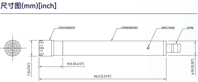
图2 CRY3401-S01 测量传声器套装尺寸图
