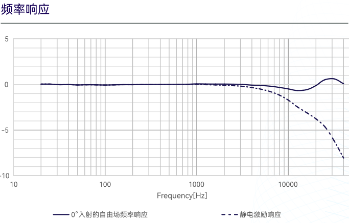
图1 CRY3401-S01 测量传声器套装典型频响曲线
