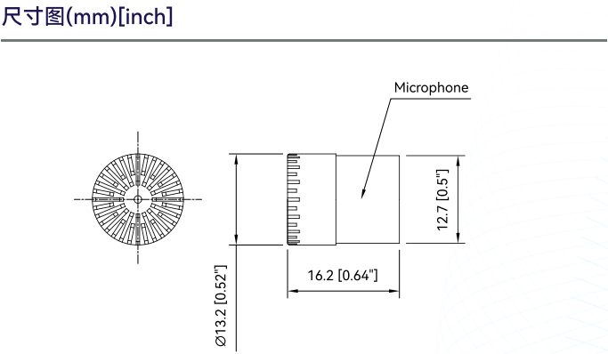
图1 CRY334 测量传声器尺寸图
