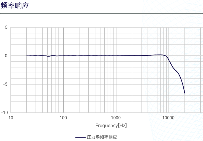
图2 CRY334 测量传声器典型频响曲线
