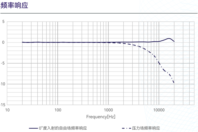
图2 CRY3285 测量传声器典型频响曲线
