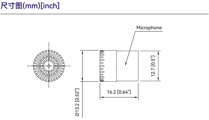
图1 CRY3285 测量传声器尺寸图
