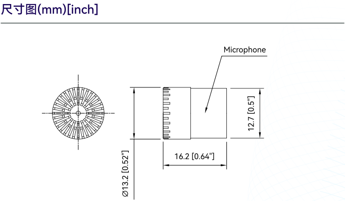
图1 CRY3204 测量传声器尺寸图
