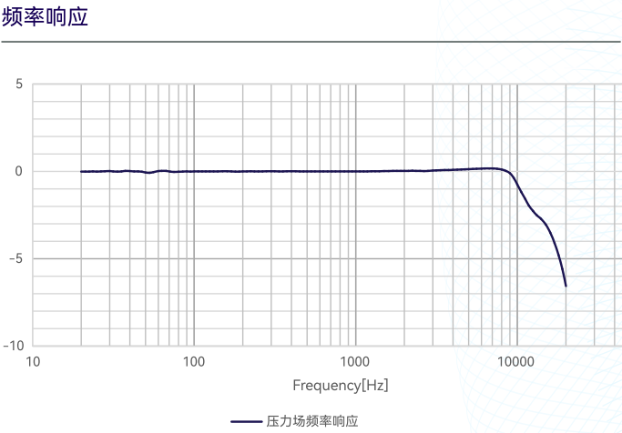
图2 CRY3204 测量传声器典型频响曲线
