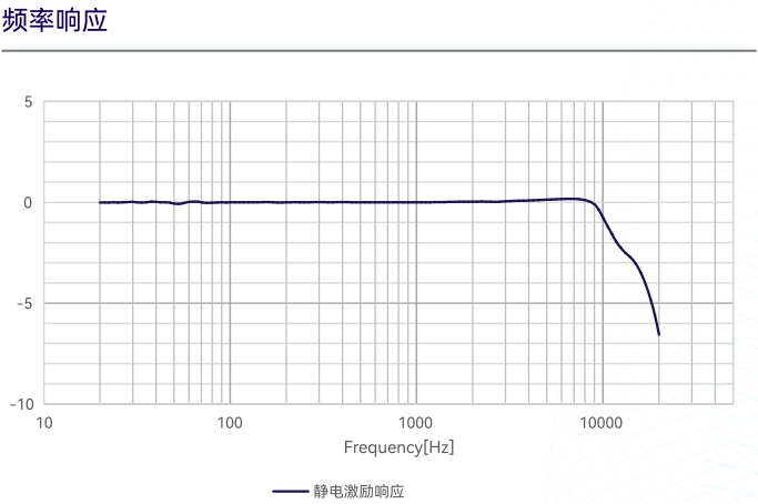
图1 CRY3204-S01 测量传声器套装典型频响曲线
