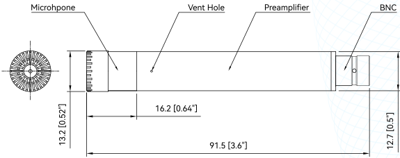
图2 CRY3204-S01 测量传声器套装尺寸图
