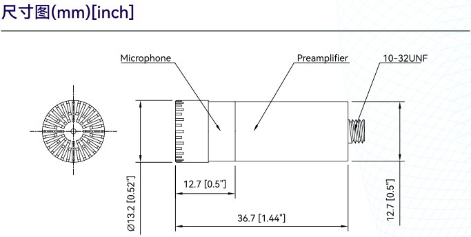
图2 CRY3202-S02 测量传声器套装尺寸图
