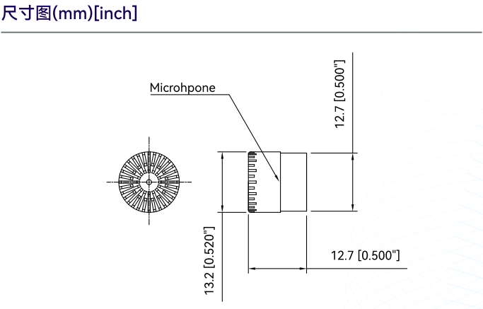
图1 CRY3201 测量传声器尺寸图
