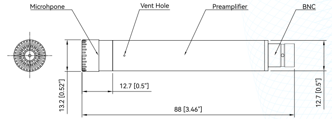
图2 CRY3201-S01 测量传声器套装尺寸图
