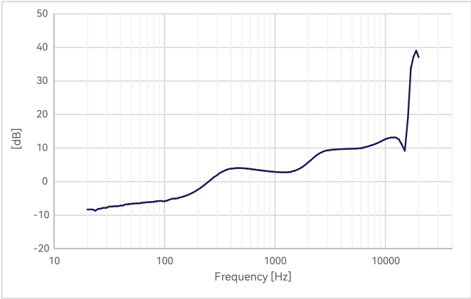
图1 CRY318 仿真耳典型频响图
