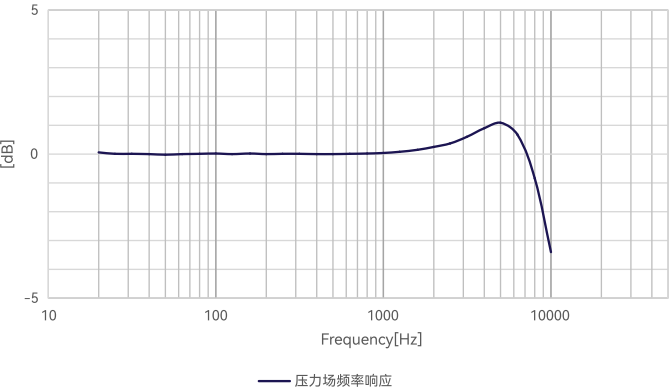
图2 CRY3102 测量传声器典型频响曲线
