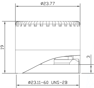
图1 CRY3102 测量传声器尺寸图
